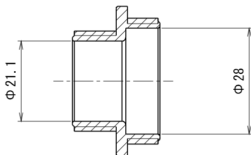
断面 A-A
